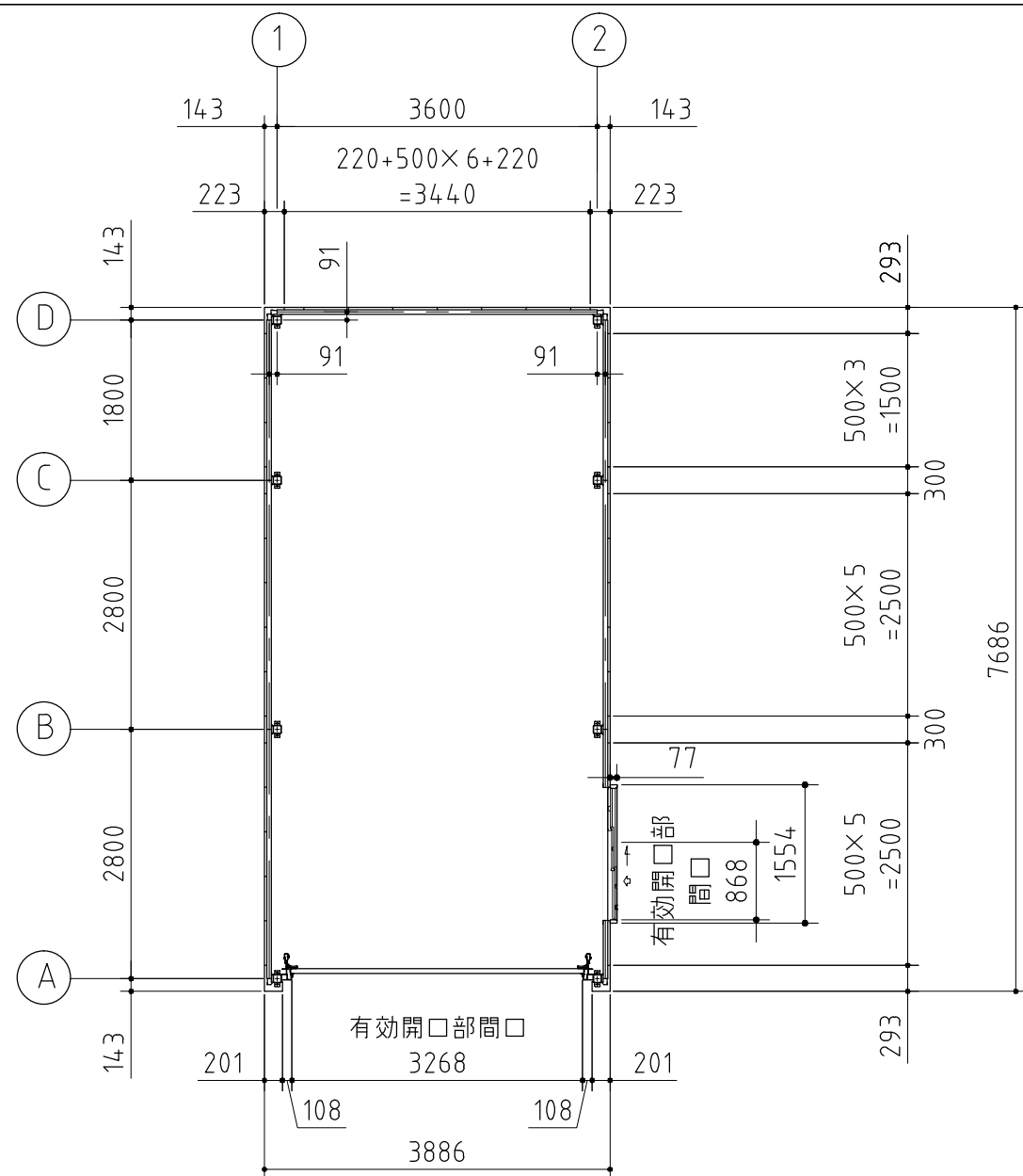
平面図
